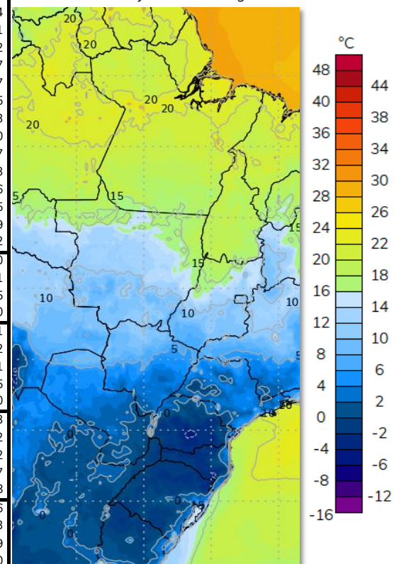
Temperaturas mínimas esperadas para o período entre 28/jul/2021 e 10/ago/2021
